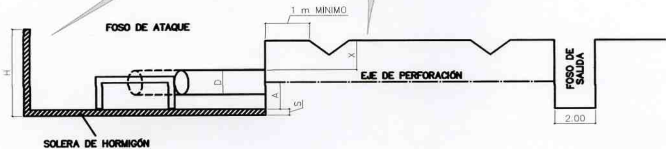
CROQUIS EN SECCIÓN
