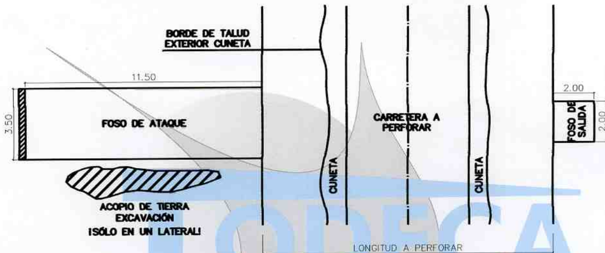
CROQUIS EN PLANTA
